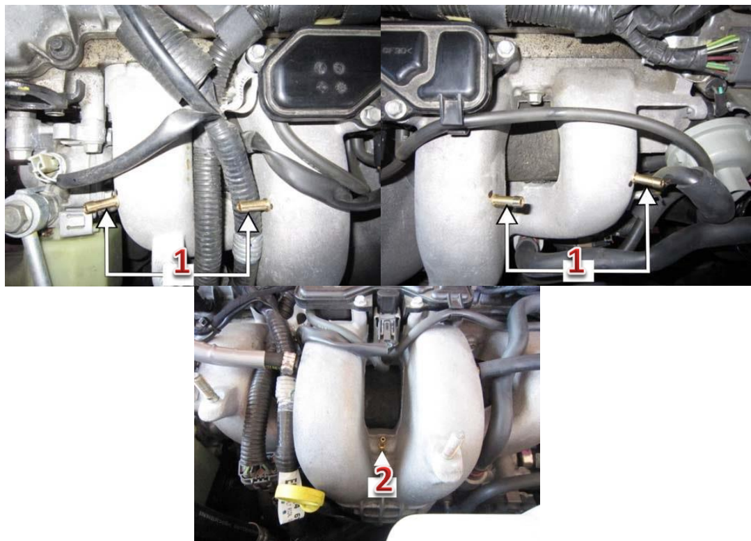
1-dysze wtryskiwaczy gazu/gas injector nozzles, 2- króciec podciśnienia/vacuum nozzle
